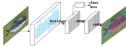
Fig. 1. Fluxograma do algoritmo de Mask R-CNN. Fonte: [1].
